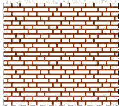
Vlaams verband in visgraat (KS0-5-2-3)
