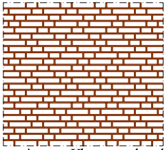
variant op Vlaams verband (KS-0-1-2-5-4-3)
