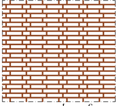
verschoven Sussexverband mit ketting (KSSS0-5)
