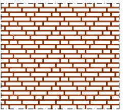
Twentsverband in visgraat (KS0-S3)
