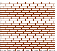
een, twee strekkenverband (S0-1-3-0-2-3-1-2)
