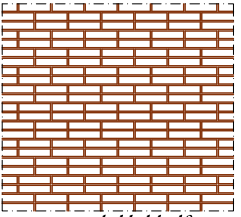
dubbel halfsteens stapelverband (S0-0-2-2)
