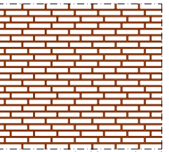
schubbverband van strekken (S0-1-2-1-0-2)
