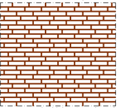
half 'kruisverband' van strekken (S0-1-0-2-3-2)
