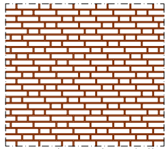
Deltrap- of Kropboller verband (KSS0-3-6-9-2-5-8-1-4-7)
