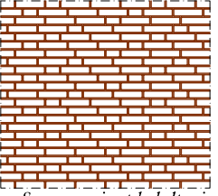
Sussex-variant kabeltrui-verband (KSSS0-3-6-9)
