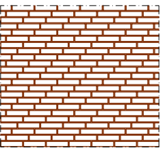
klezorenverband met vallende tand (S0-1-2-3)
