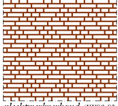
vlechtwerkverband (KKS0-S3-KKS4-KKS5-KKS6-S3-KKS2-KKS1)
