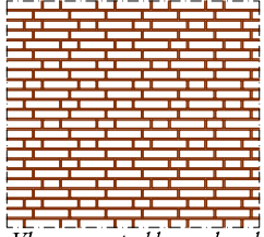
Vlaams en strekkenverband (KS0-S3-KS2-S3-KS4-S3)
