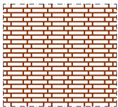
Noors kettingverband (KSS0-5)
