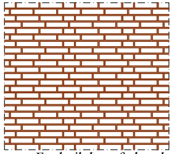
DK: Frederiksberg forbandt (KSS0-S1-KSS0-K3)
