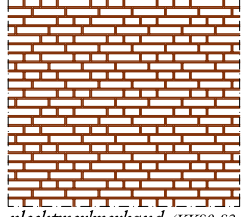
vlechtwerkverband (KKS0-S3-KKS4-S1-KKS6-S3-KKS2-S1)
