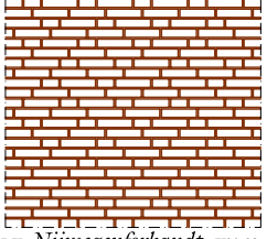
DK: Nijmegenforbandt (KS0-S3-KS4-S1-KS0-S3-KS2-S1-KS4-S3-KS2-S1)
