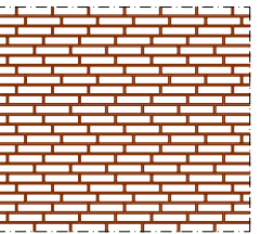
grote zigzag (S0-1-2-3-2-1)
