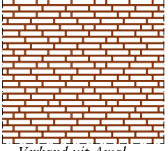
Verband uit Amal (KS0-S3-KSS5-KSS0-KSS5-KKKS8-KKKS3-KSS0-KSS5)
