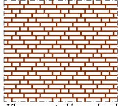
Vlaams en strekkenverband (KS0-S1-KS2-S3-KS4-S1-KS0-S3-KS2-S1-KS4-S3)
