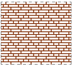
frans verb. en strekkenlaag visgraat (S0-KKS7-S2-KKS3)
