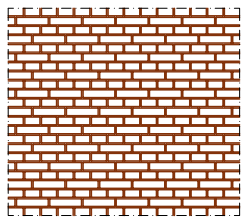
kruisverband (K0-S1-K0-S3)
