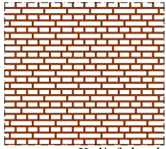
DK: Koch's forbandt (K0-S1-K0-S1-K0-S3-K0-S3)
