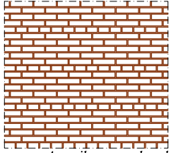
Amerikaans verband (K0-S3-1-3-1-3)
