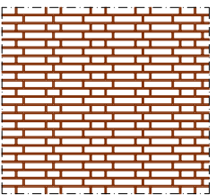
Twents kettingverband (KS0-S3)
