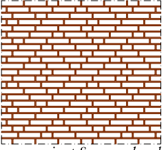
variant Sussexverband (KSSS0-7-2-9-0-1-6-13-8-1-6-7-12-5)
