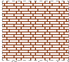
Vlaams en kruisverband (KS0-S1-KS0-S3)
