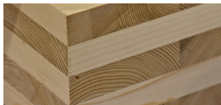
Figuur 36. CLT detail
