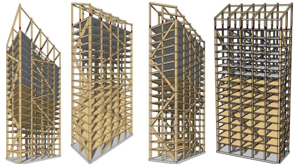
Figuur 37. CLT constructie Mjösa toren (Voll Arkitekter)
